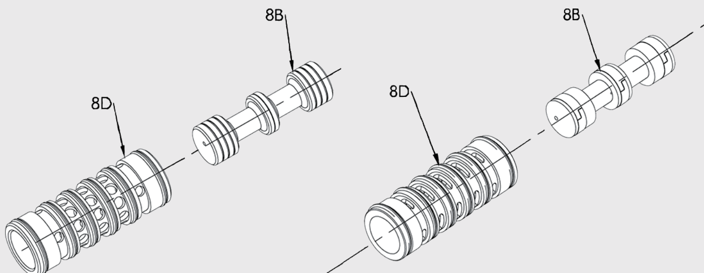
LISTA DE PIEZAS DEL KIT DE REPARACIÓN DEL PISTÓN DE LA CHAQUETA
