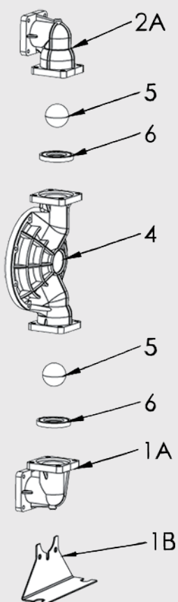
CUERPO PLÁSTICO
