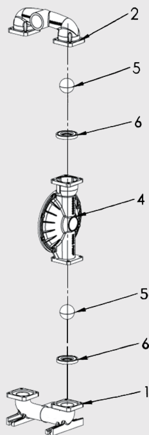
CUERPO METÁLICO
