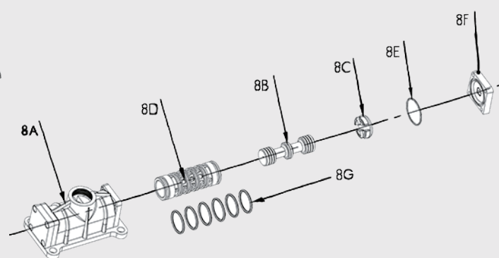
LISTA DE PIEZAS DEL KIT DE REPARACIÓN DE LA VÁLVULA DE AIRE (CUERPO DE METAL)
