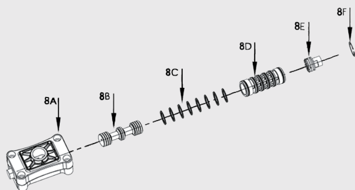
LISTA DE PIEZAS DEL KIT DE REPARACIÓN DE LA VÁLVULA DE AIRE (CUERPO DE PLÁSTICO)
