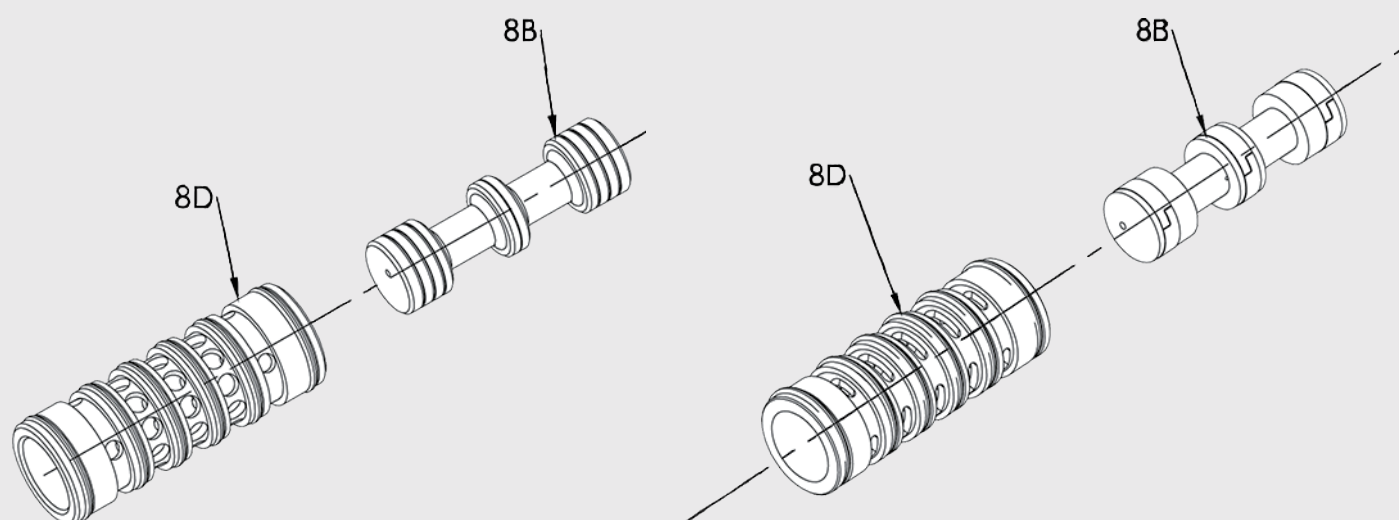
LISTA DE PIEZAS DEL KIT DE REPARACIÓN DEL PISTÓN DE LA CHAQUETA
