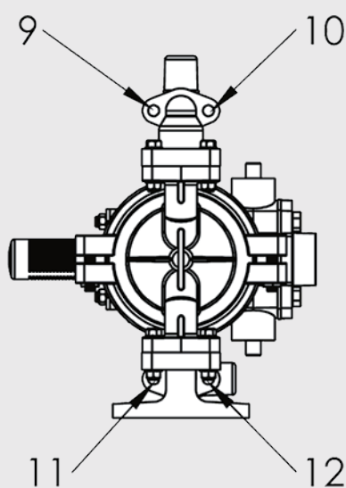
TAPA DE LÍQUIDO DERECHA IZQUIERDA Apriete los tornillos con un par de 6N.m_10N.m
