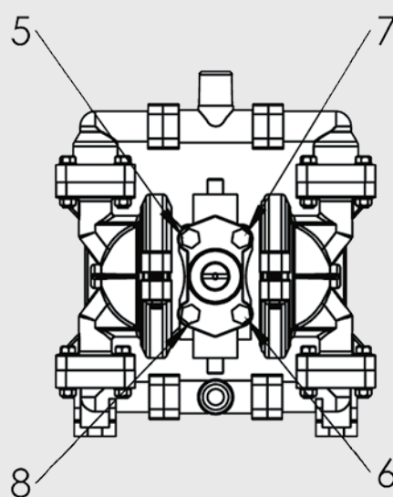
CUBIERTA DE VÁLVULA PILOTO Apriete los tornillos con un par de 6N.m_9N.m
